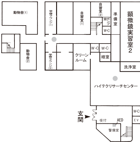
3階
